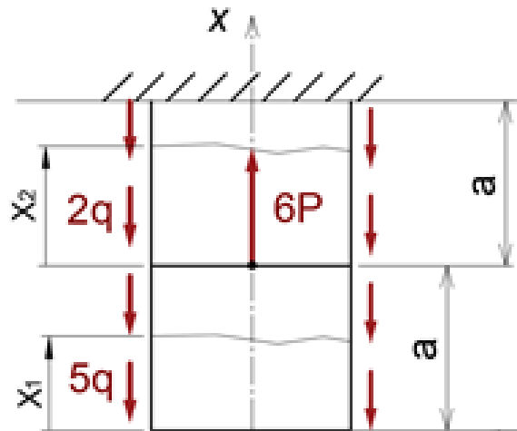
Рис. 1- Расчетная схема нагружения бруса.
